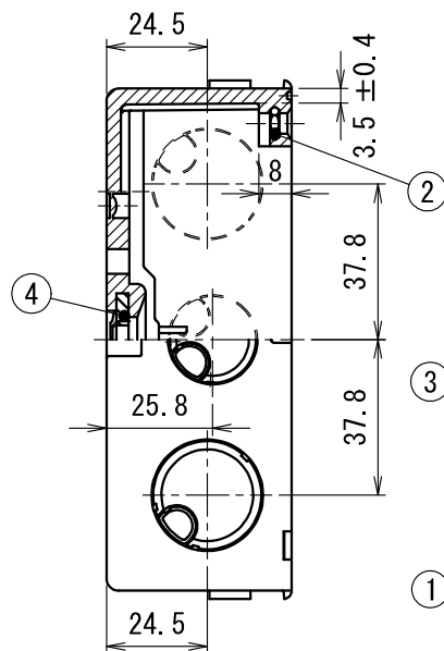
A-A 断面図
